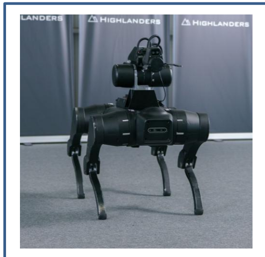
<四足歩行ロボット：HLQ Edge>
