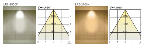
LR6-3500K LR6-2700K 白熱電球100W相当
